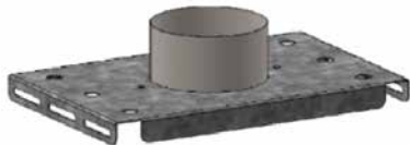
Jalustan pohjalevy, jonka pohjassa on puhdistusluukku.
